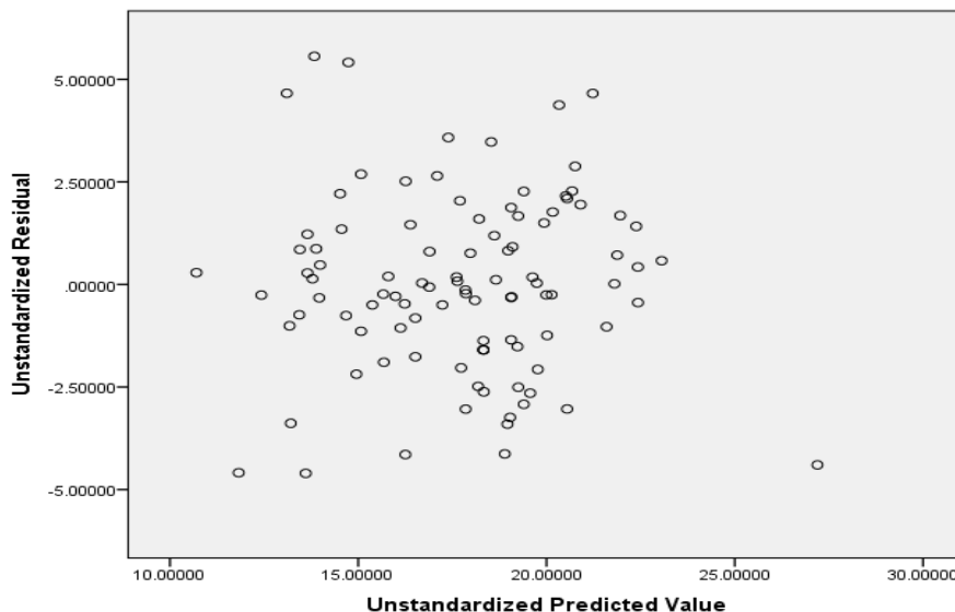
Gambar Grafik Scatter Plot Hasil Uji Heteroskedastisitas
